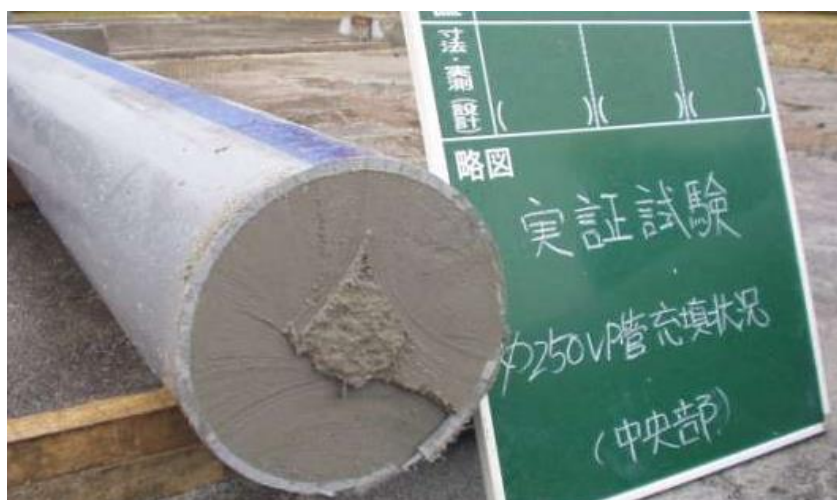
セルクリート工法による管内充填状況 実証試験施工による確認
